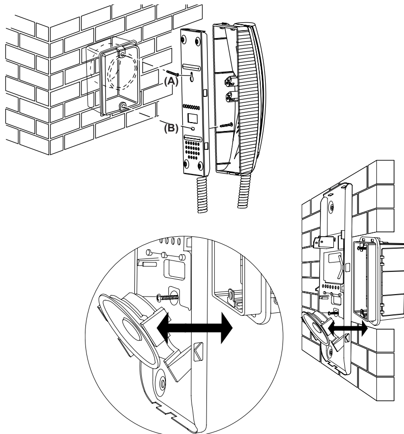
Fig. 2 Installazione a parete • Wall mounting Montage mural • Aufputzmontage Sujección ed pared • Instalação na pared
