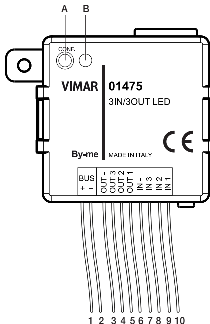
VISTA FRONTALE - FRONT VIEW - VUE DE FACE VISTA FRONTAL - FRONTANSICHT - ΜΠΡΟΣΤΙΝΗ ΠΛΕΥΡΑ
